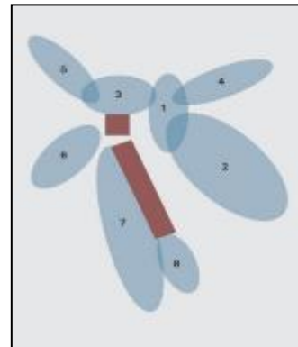
Εικόνα 13: «Νεκρές γωνίες» οδηγού φορτηγού σε συγκεκριμένη θέση ελιγμού.
